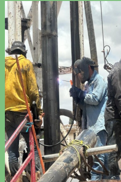
CONTINÚA LA PERFORACIÓN E INSTALACIÓN DE TUBERÍA EN EL POZO DE LA COMUNIDAD DE BIMBALETES
